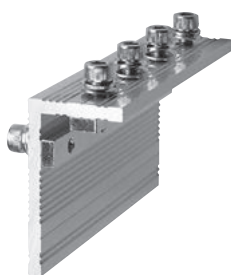
品名 連結キット 型式 ARS050A-CN1
