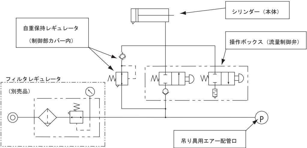
＜「けんすい」本体エア回路図＞
